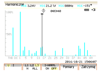
Rysunek 5. Wykres harmonicznych
