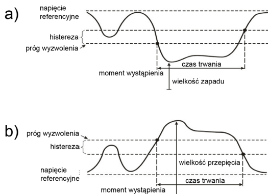
Rysunek 4. Graficzna definicja zapadów i przepięć
