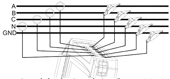
Rysunek 1. Napięciowe i prądowe gniazda analizatora SA2100
