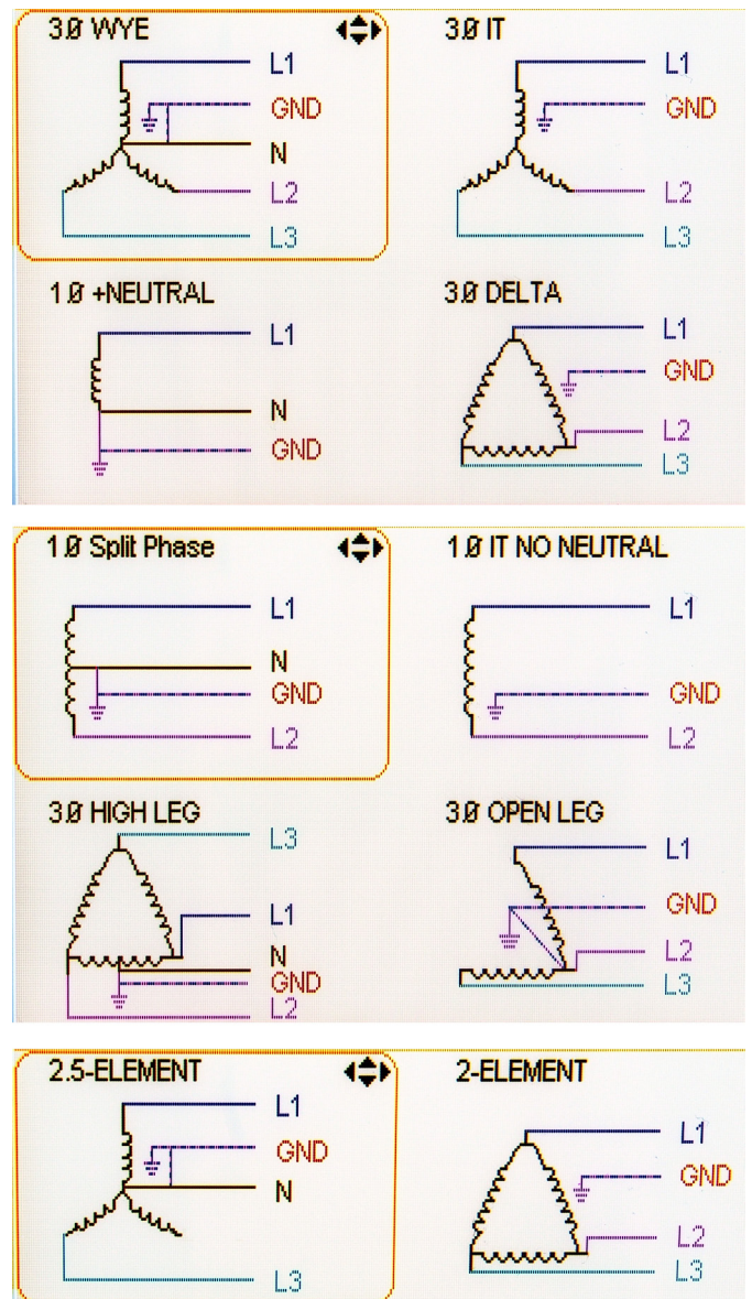
Rysunek 2. Konfiguracje sieci mierzonych analizatorem SA2100
