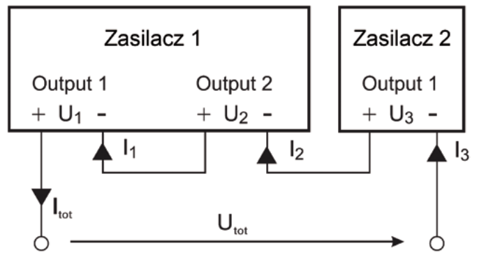
Rysunek 6. Szeregowo połączenie zasilaczy
