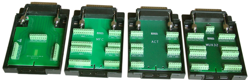
Fotografia 3. Moduły połączeniowe
