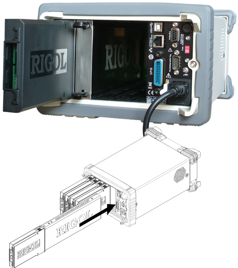
Fotografia 4. Widok jednostki centralnej M300 od tyłu – ilustracja zasady instalowania kart
