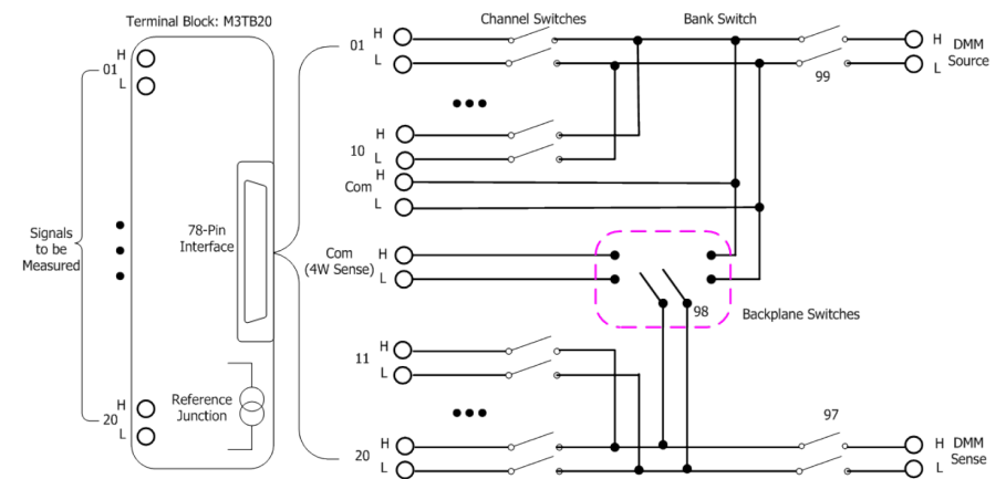
Rysunek 6. Schemat połączeń realizowanych przez kartę MC3120
